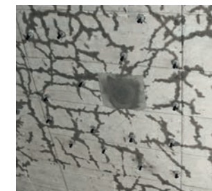
Rissverpressung
